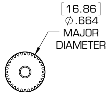
10:1 PLANET GEAR 32T
