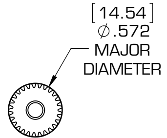
5:1 PLANET GEAR 27T
