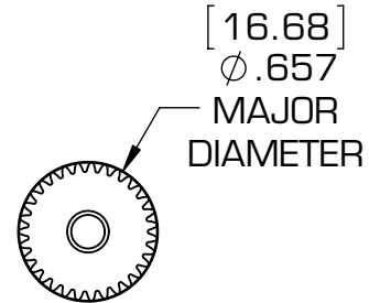
9:1 PLANET GEAR 31T
