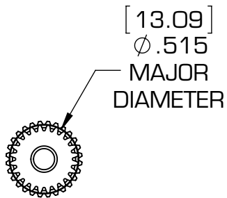
4:1 SUN GEAR 24T
